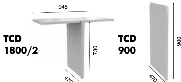
Перегородка вертикальная
