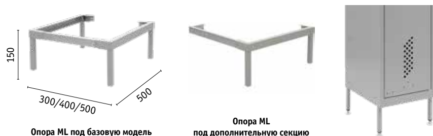
Опора ML под базовую модель
